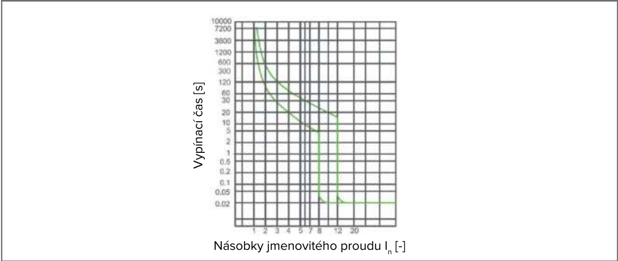
Vypínací charakteristika
