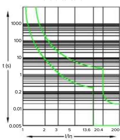
Charakteristika K
