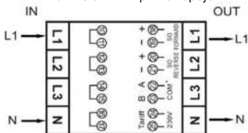
Ex9EMS 3P 4M - přímé zapojení - 1P 2W - jedna fáze
