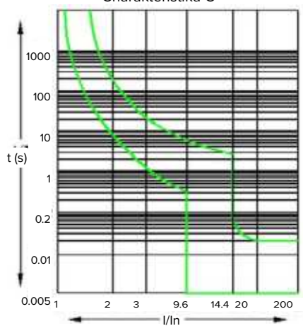
Charakteristika C
