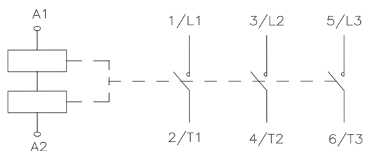
Schéma zapojení
