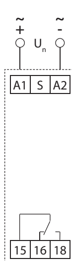
Ex9TR C - Ciclor începând cu puls
