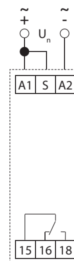
Ex9TR C - Ciclor începând cu pauză
